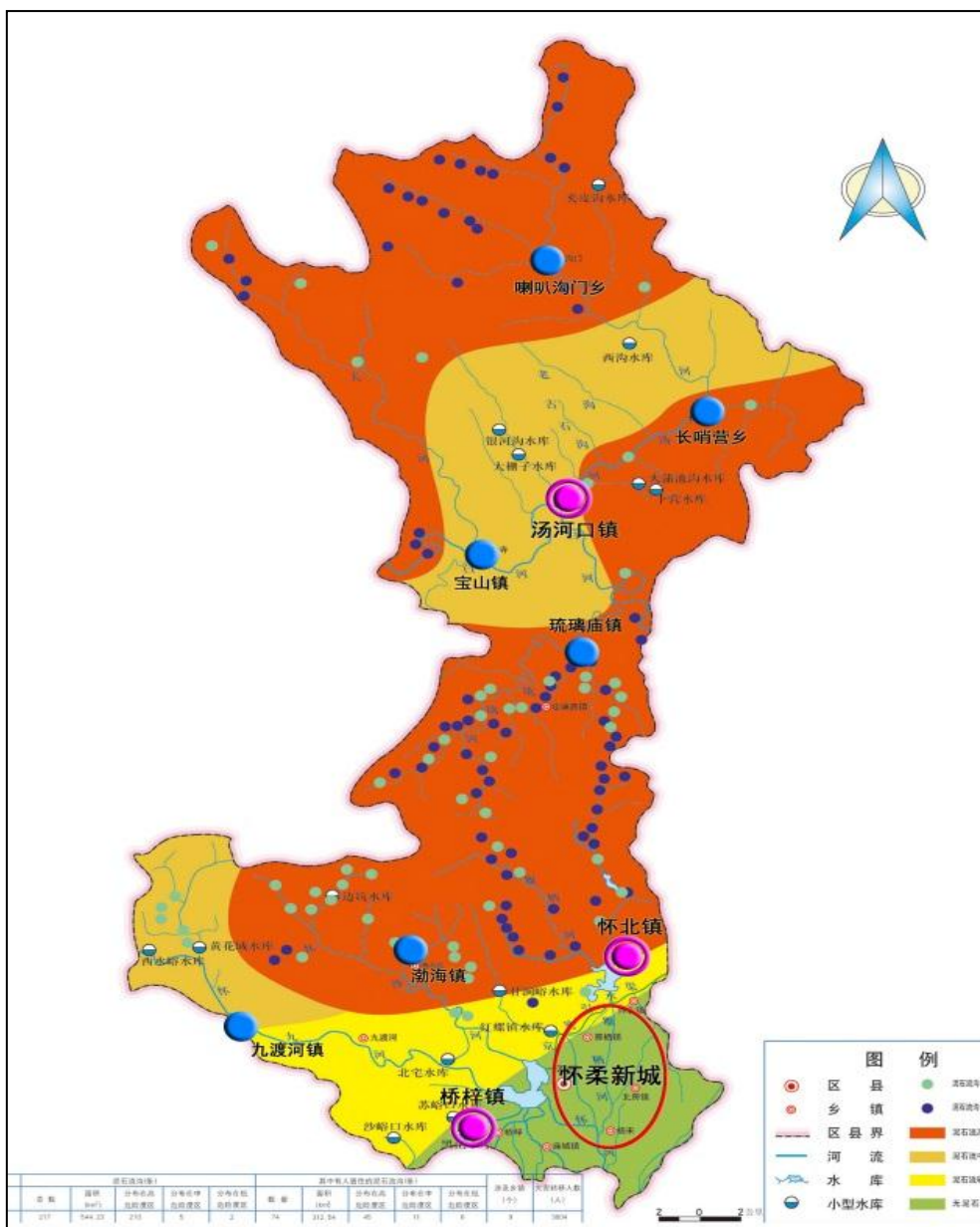
图 6-8 “十三五”期间怀柔区防洪防灾工程图
